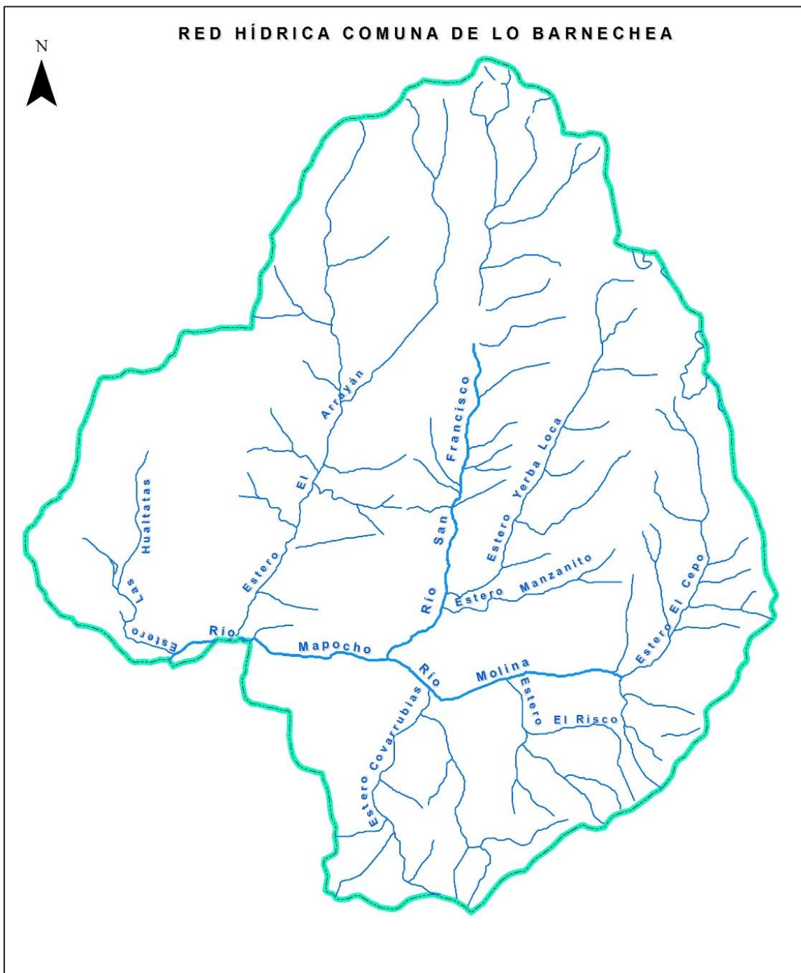
IMG 04: Red Hídrica de la Comuna de Lo Barnechea. Fuente: Elaboración propia.
